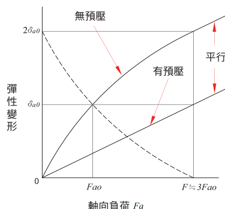
圖4.4.1.5 彈性變形曲線
