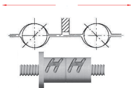
圖4.4.1.1 伸張預壓
