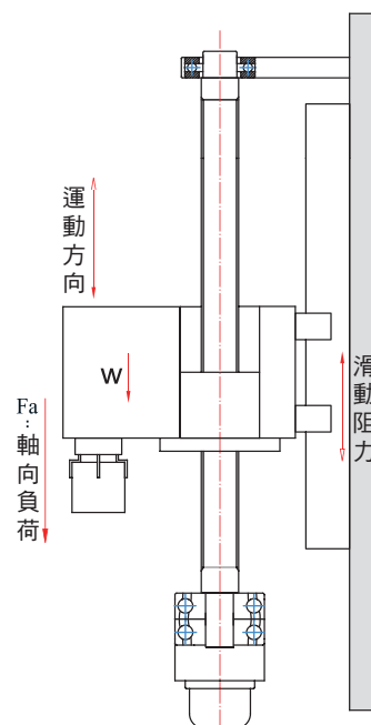
垂直搬運裝置
