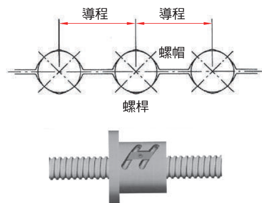
圖4.4.1.2 四點接觸預壓
