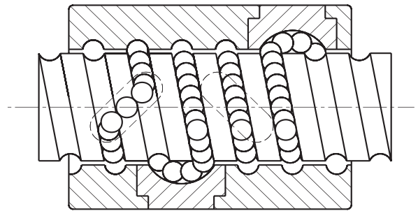
圖4.3.1.4 內循環螺帽圖
