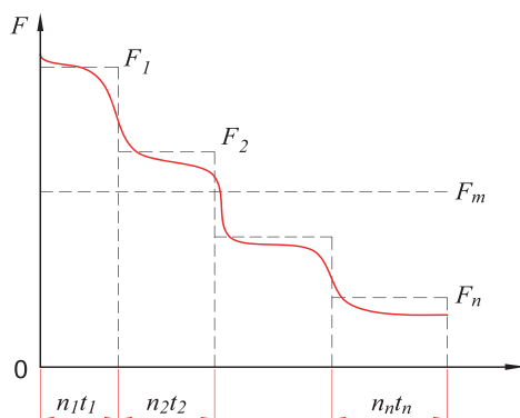
圖4.5.2.1 階段變動負荷
