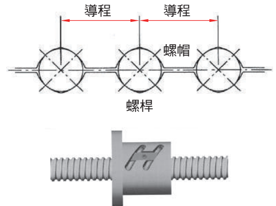
圖6.4.1.2 四點接觸預壓
