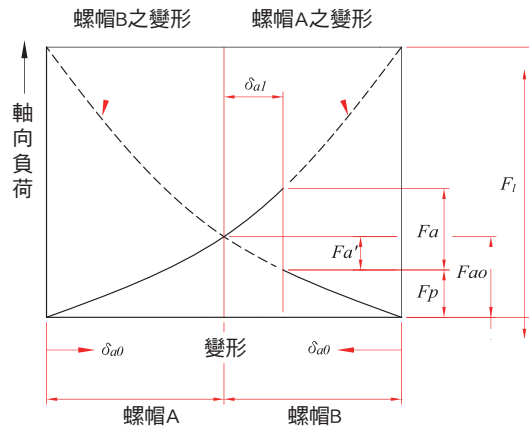
圖6.4.1.4 定位預壓變形關係圖
