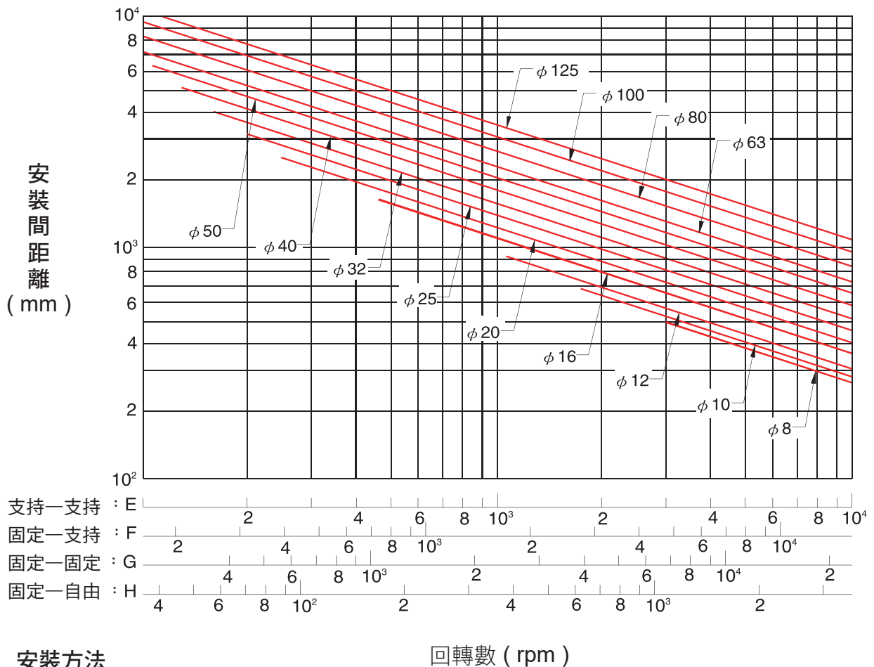
圖6.2.3.1 軸對於危險速度之容許轉數
