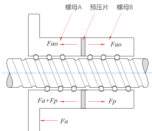
图6.4.1.3 双螺母之定位预压
