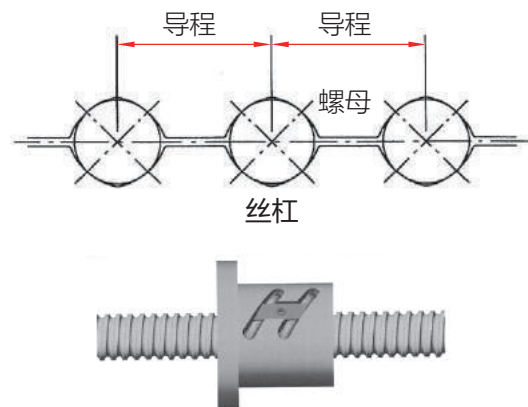
图6.4.1.2 四点接触预压
