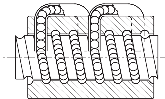
图6.3.1.2 外循环螺母图
