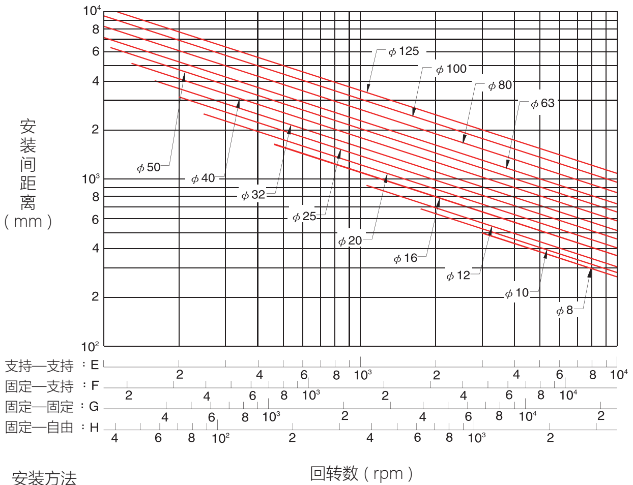
图6.2.3.1 轴对于危险速度之容许转速
