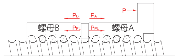
图6.3.2.1 双螺母预压负荷
