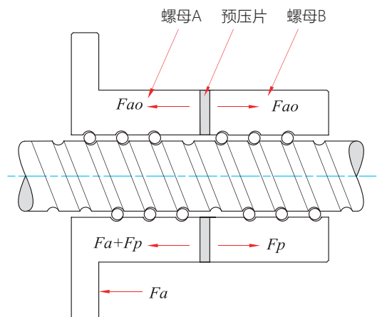
图6.4.1.3 双螺母之定位预压
