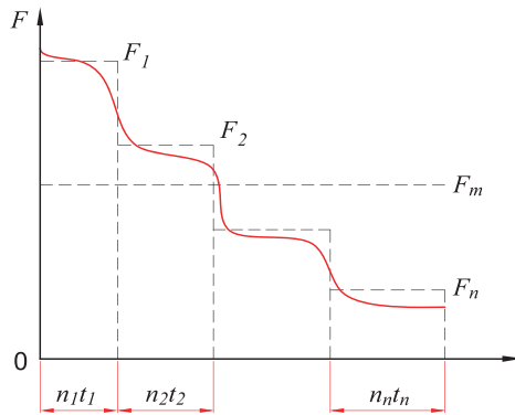
图6.5.2.1 阶段变动负荷
