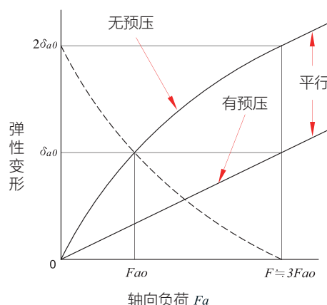
图6.4.1.5 弹性变形曲线
