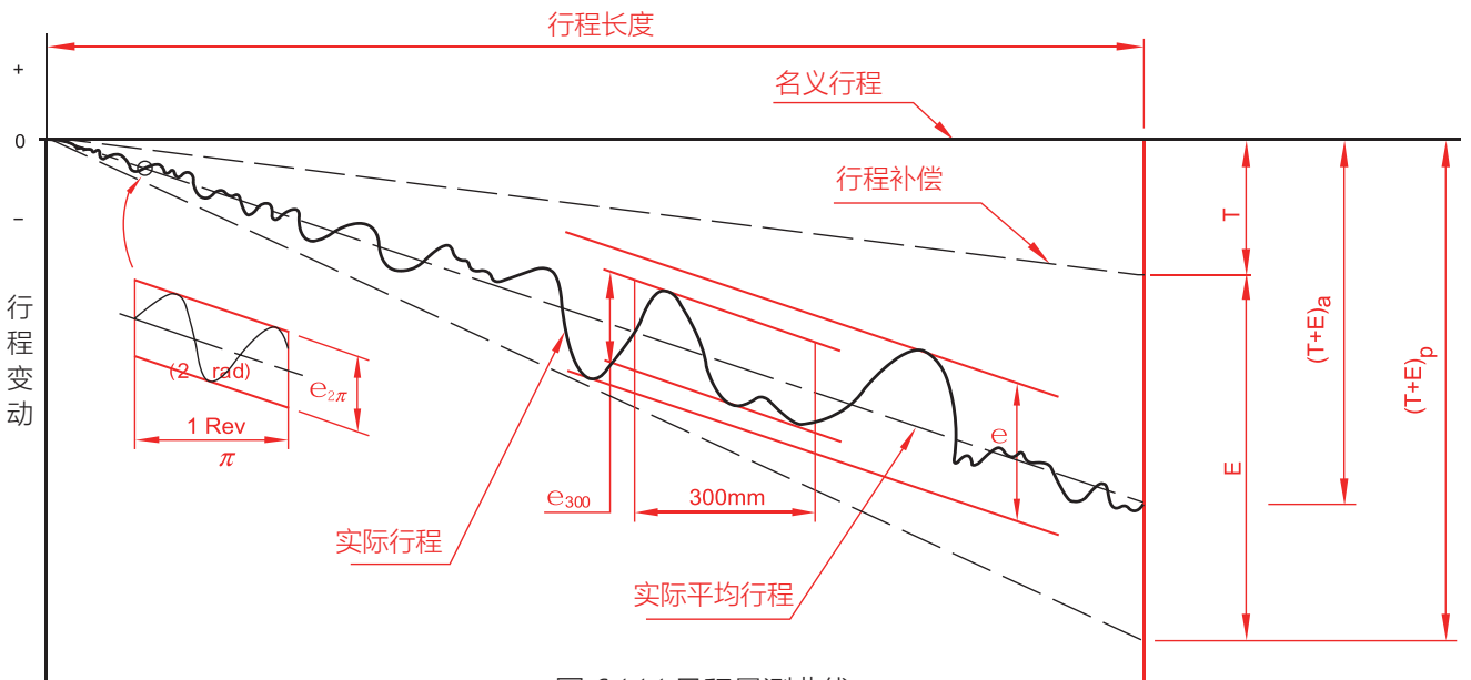
图 6.1.1.1 导程量测曲线
