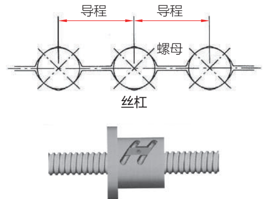
图6.4.1.2 四点接触预压
